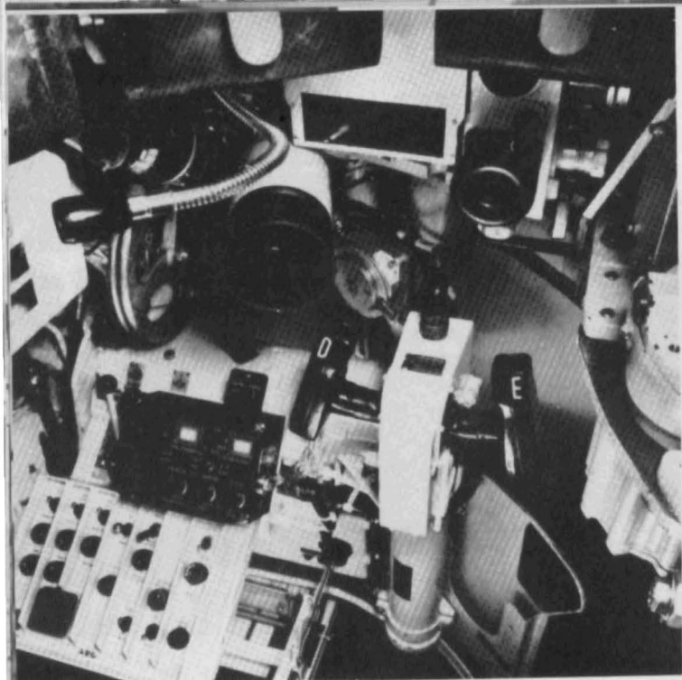
Richtschützenplatz mit Okular des WBG-X in Bildmitte. Rechts unterhalb davon der Doppelrichtgriff mit Kliniken für Dauer- (D) und Einzelfeuer (E). Links unten das Bedienpult. (Zeiss)
