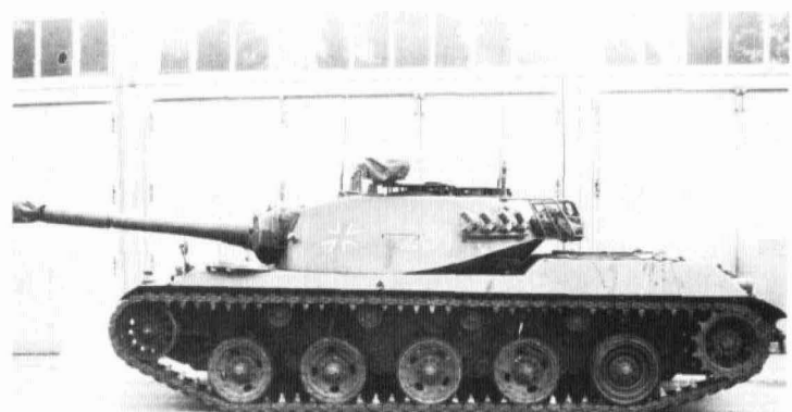
1967/68 übergab die Industrie 300 Jagdpanzer, Rakete der neuen Baureihe (Panzerabwehrenkrakete SS 11 / vier Mann Besatzung) der Bundeswehr.
