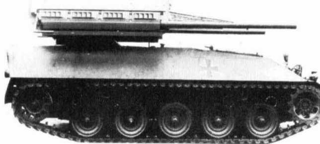
Prototyp RU 242, Raketenwerfer mehrfach leicht (90 mm-Raketen) Oerlikon der Fa. Hanomag. Dieses Fahrzeug wurde 1967 als Erprobungsträger "RO-LAND" umgebaut.
